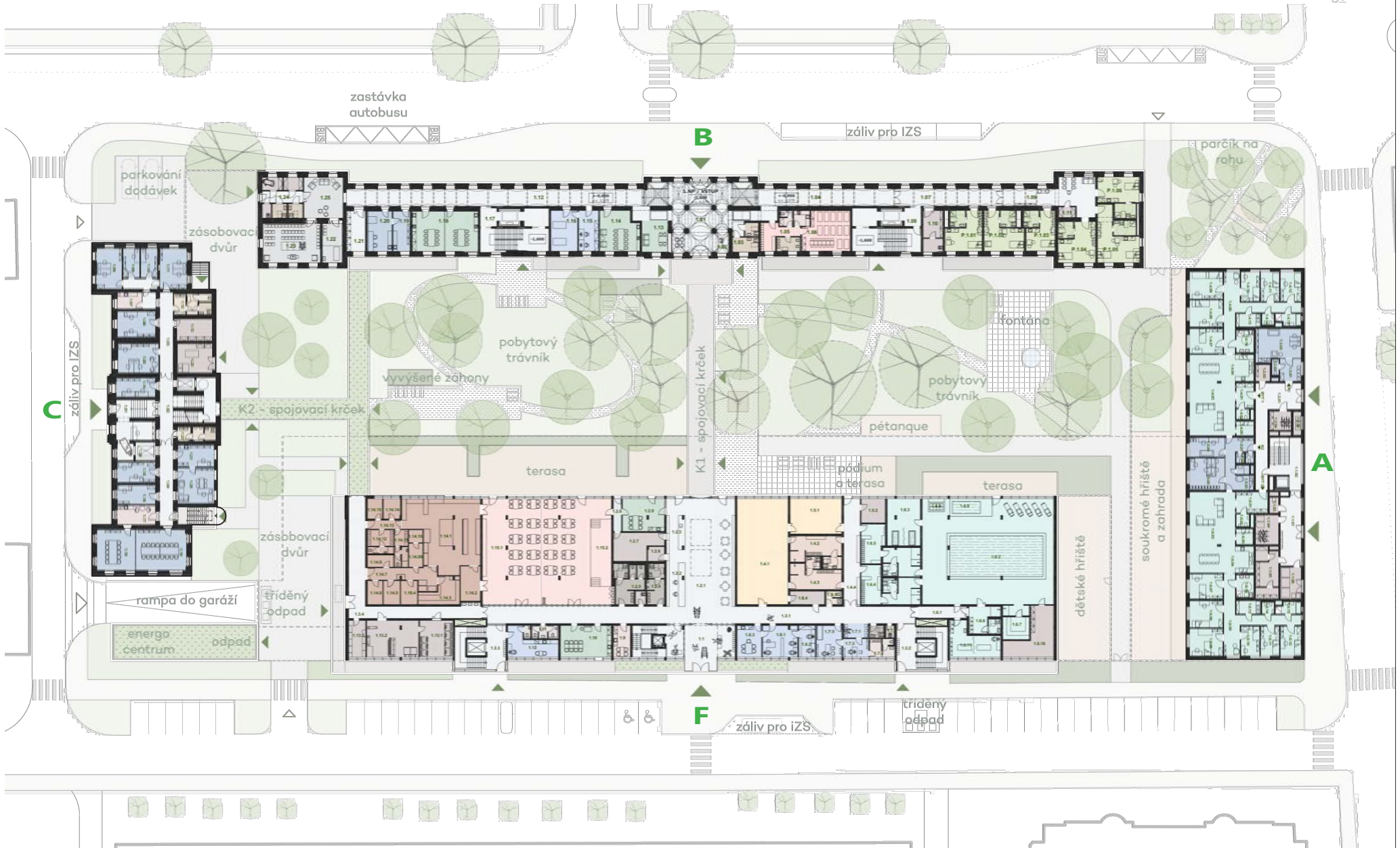
půdorys na úrovni přízemí
